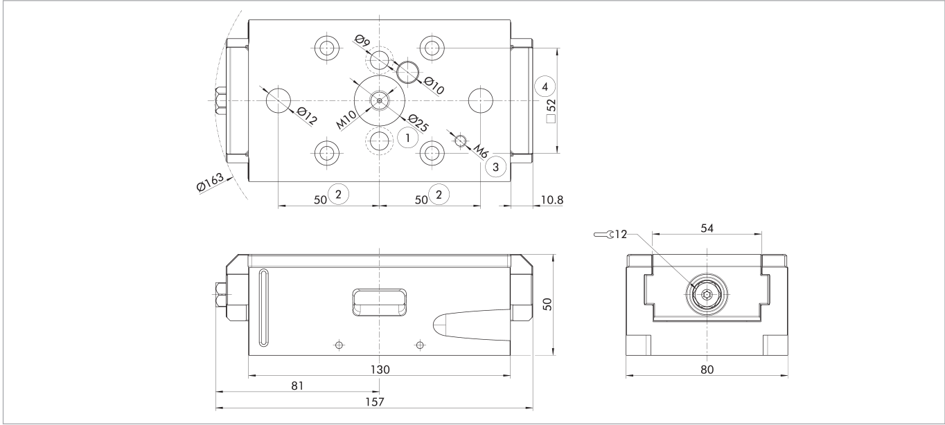
① NSE3クランプングピンに対応 ② インデックスピンに対応 ③ クランプングデバイスを正しく位置合わせするためのボカヨケボア穴 ④ GFD-SP mini Ø16 h6 クランプングピンに対応
